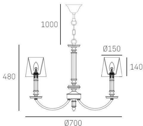
WYMIARY
